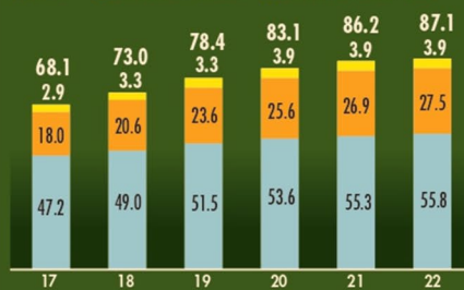
*/ Sistema Interconectado Nacional **/ Sistema Eléctrico Nacional FUENTE: ELABORACIÓN PROPIA CON DATOS DEL PRODESEN (DIVERSOS AÑOS)
